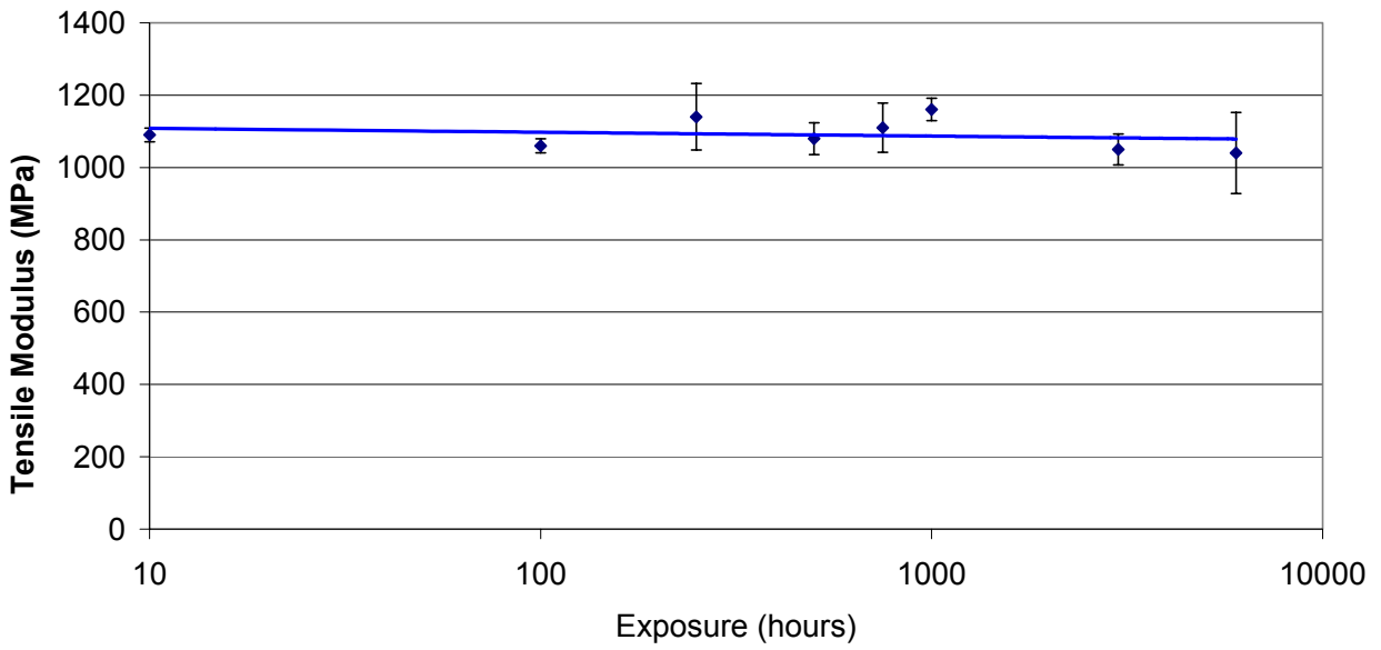
Tensile Modulus: PP Bumper
