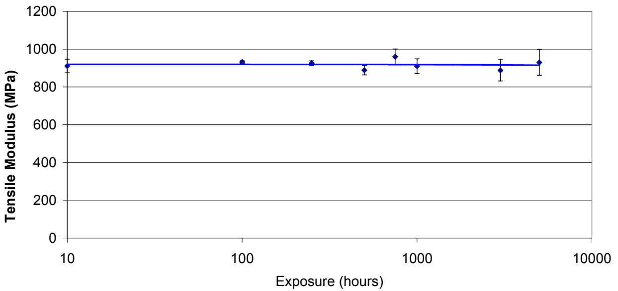
Tensile Modulus: Wheelie Bin Black
